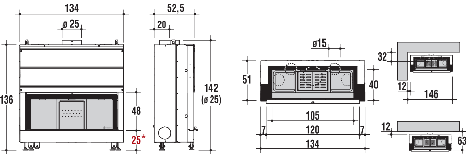
LIGHT 06N à bois à air chaud convection naturelle
