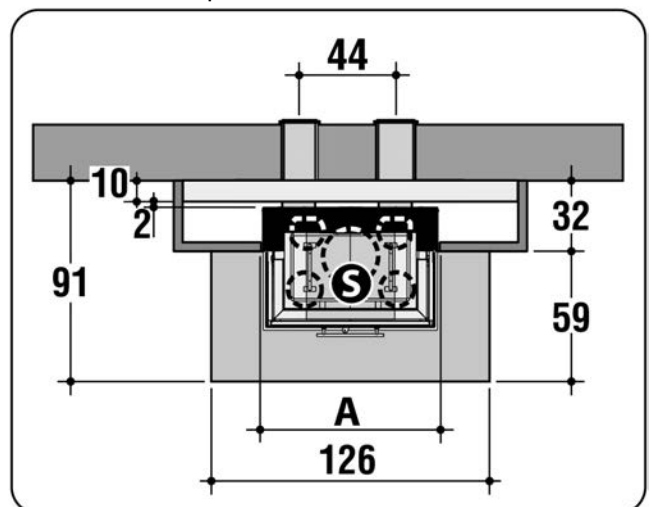
avec kit canalisation air convection naturelle (2 su 3 prise d'air extérieur Ø 15 cm)
