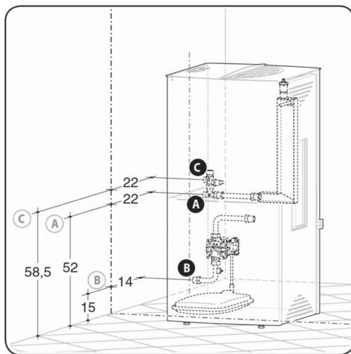
A. Arrivée à l'installation (3/4" m) B. Retour à l'installation (3/4" m) C. Vidange soupape de sécurité (1/2" f - 3 bar)
